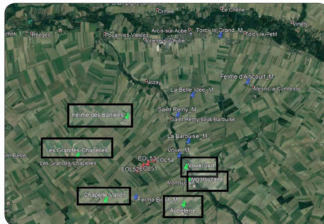
Récepteurs des calculs, modélisation du site avec futures éoliennes du projet (en rouge) : points complémentaires (en vert et encadrés) et points de mesures (en bleu), extrait de l'étude d'impact acoustique, ECHOPSY, 2020
