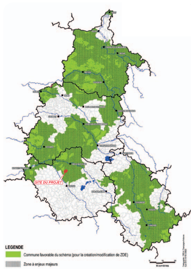
Zones favorables au développement de l'énergie éolienne et contraintes (SRE de Champagne-Ardenne)
